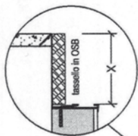
Particolare Battuta persiana con lamiera zincata e tassello in OSB
